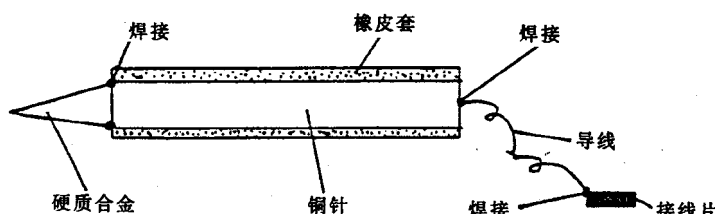
图 1 测量探针
